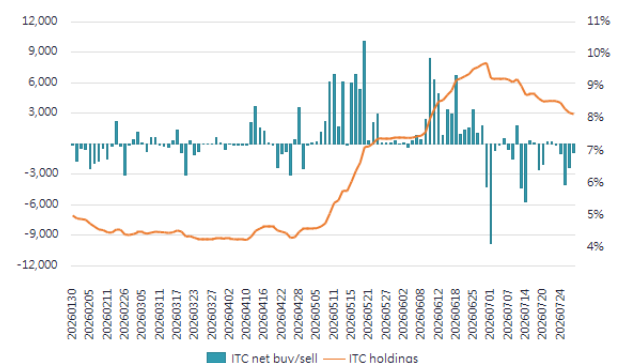
圖表 11：投信買賣超張數及持股比率
